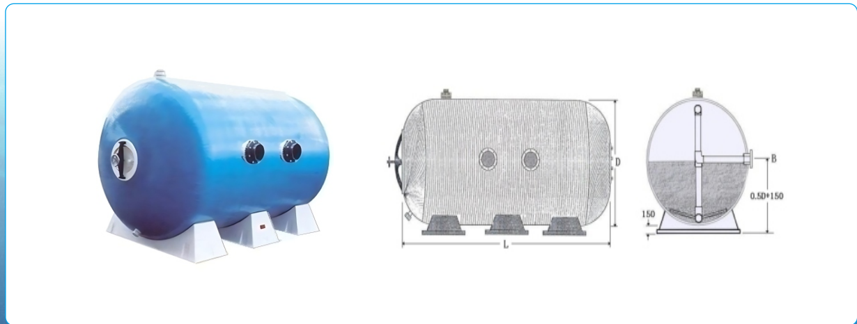
FH臥式過濾砂缸
